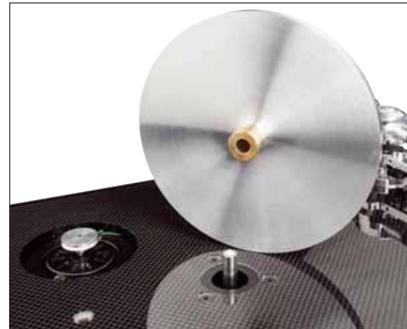
Der in den Unterbau eingelassene Motor mit Lager und Subteller
